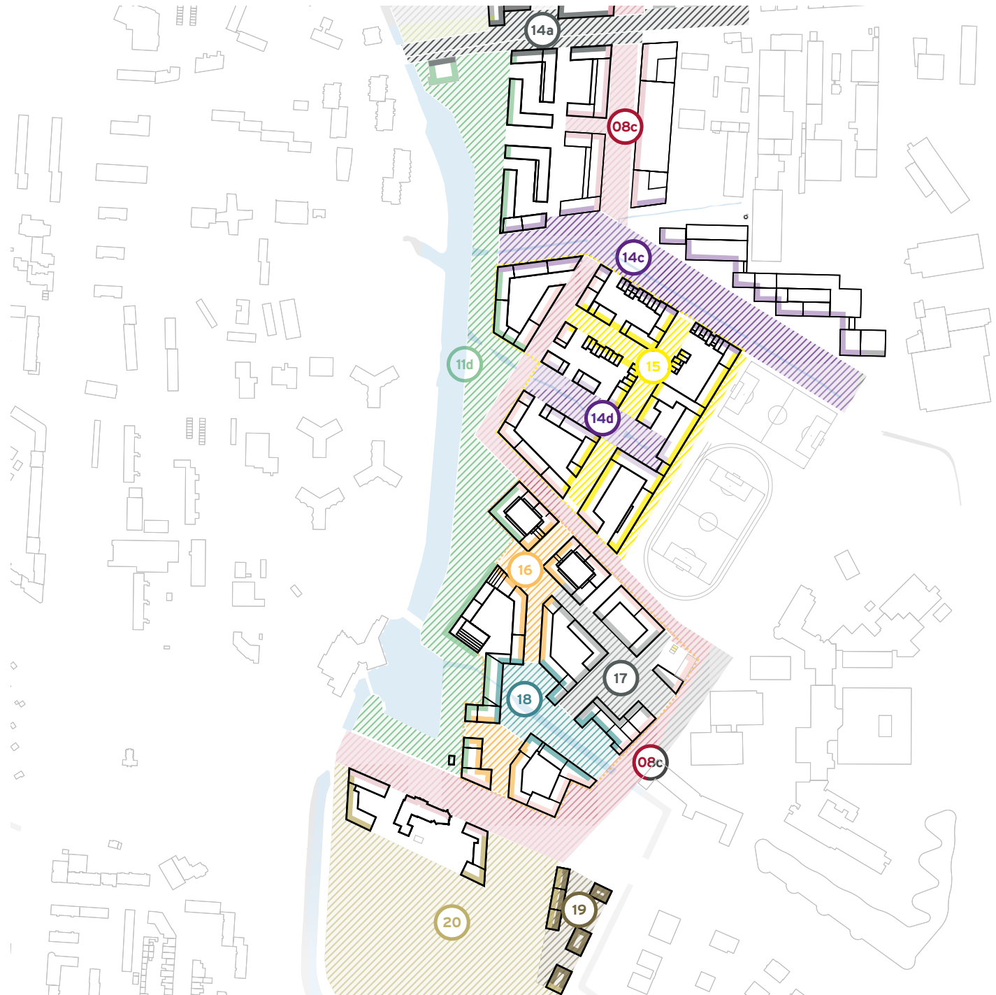
Abb. 217: Lagen des Wilhelmsburger Rathausviertels
