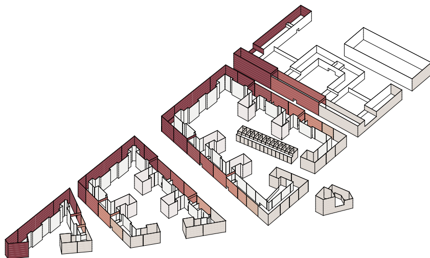
Abb. 132: Isometrische Darstellung des Farbkonzepts
