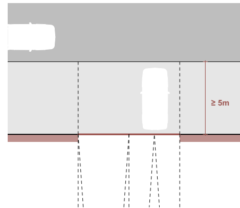
Abb. 111: Schema-Grundriss bündige Tore
