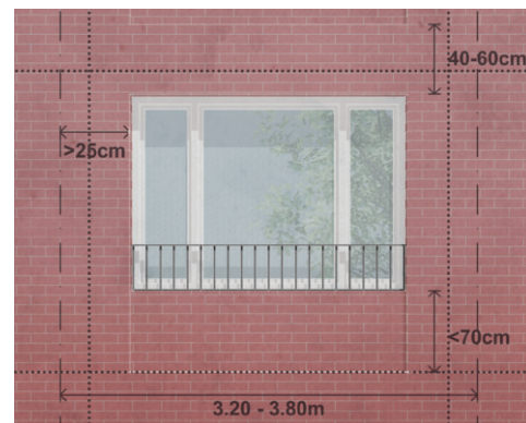
Abb. 138: Öffnungsproportion mit massiver Brüstung
