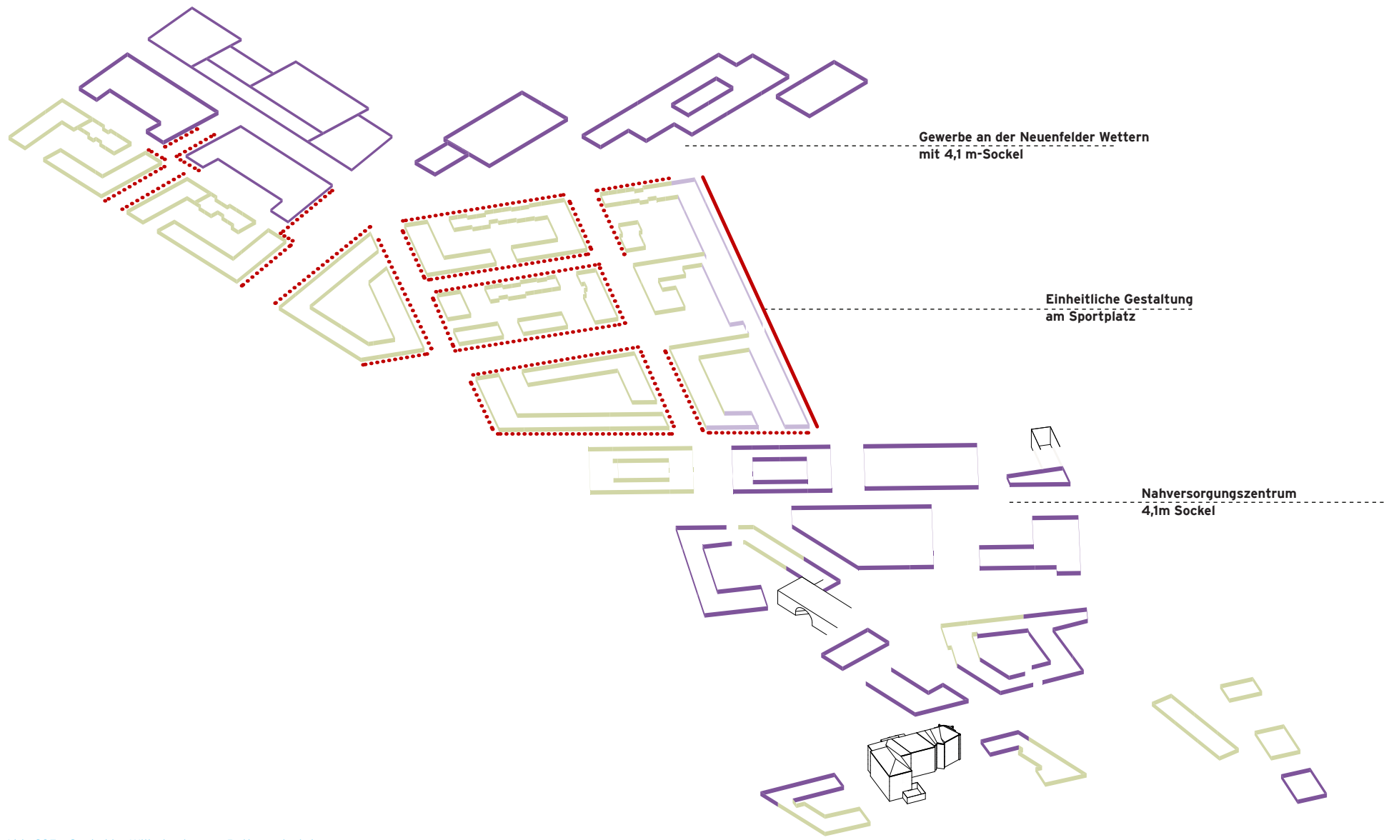
Abb. 235: Sockel im Wilhelmsburger Rathausviertel
