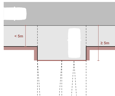
Abb. 111: Schema-Grundriss bündige Tore
