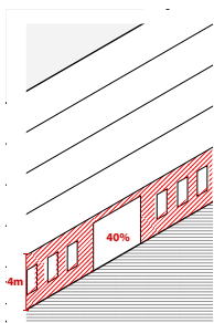
Abb. 150: Sockelregeln
