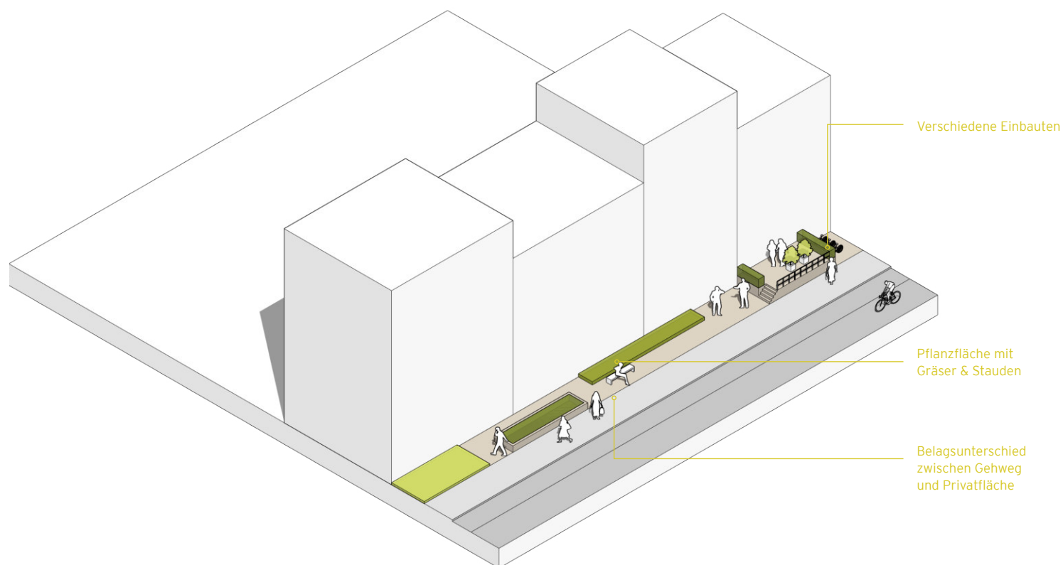
Abb. 83: Isometrie der offenen Vorzone
