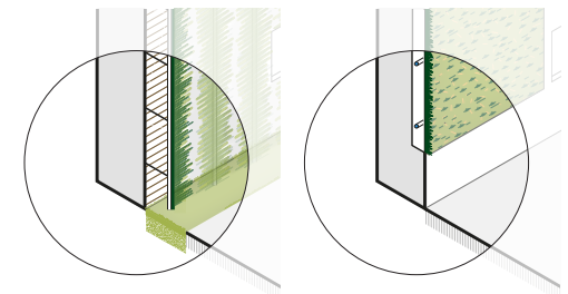
Abb. 48: Schema bodengebundenen System
