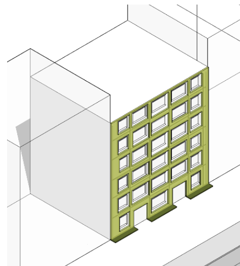
Abb. 49: Axonometrie bodengebundenen System
