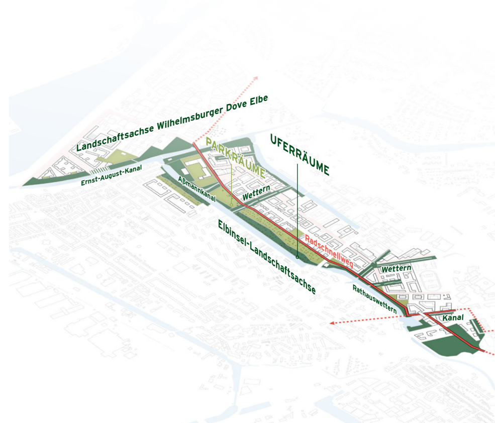
Abb. 09: Übersicht der Uferräume
