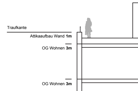
Abb. 66: Beispiel Dachabschluss Traufkante
