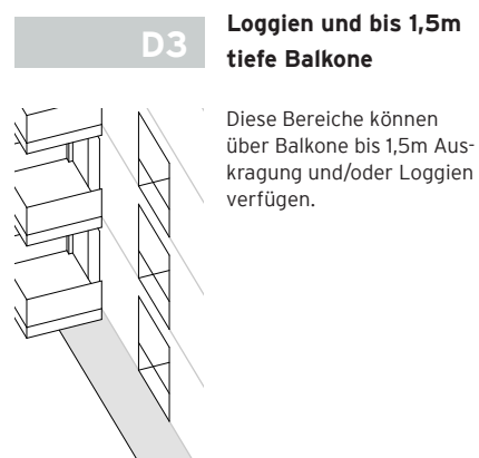
Abb. 202: Regeln Balkone und Loggien
