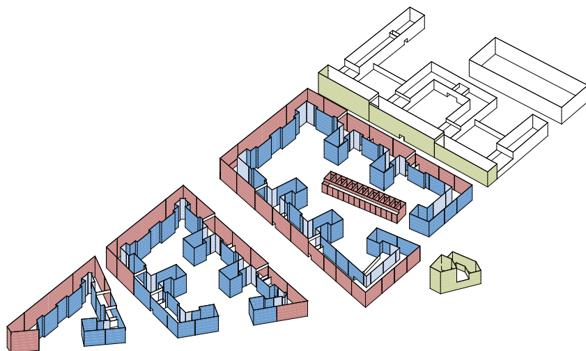
Abb. 159: Isometrische Darstellung der Verortung der Balkone und Loggien
