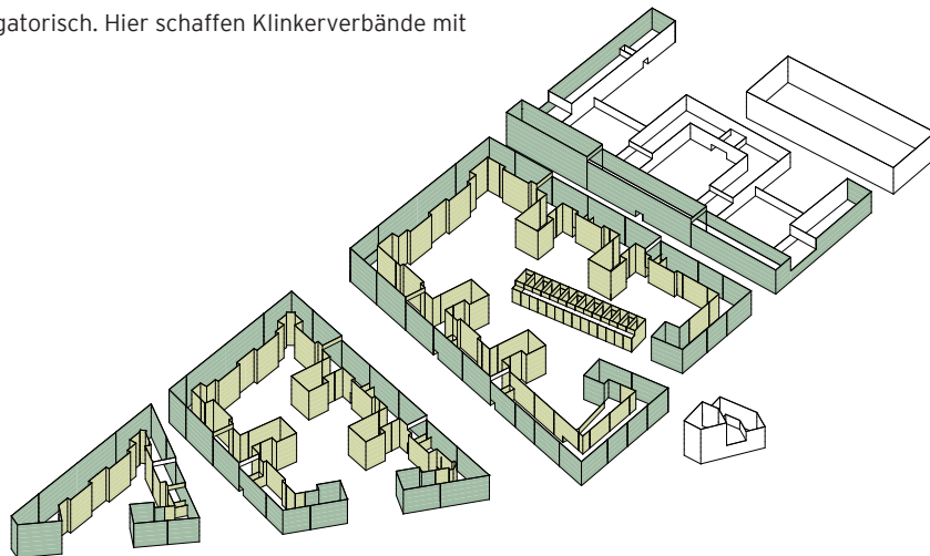
Abb. 142: Isometrische Darstellung der Verortung des abgesetzten Sockels
