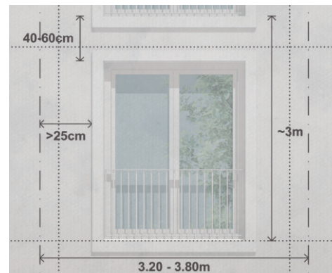
Abb. 137: Öffnungsproportion beim bodentiefen Fenster
