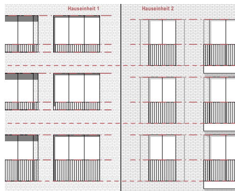
Abb. 136: Anordnung der Öffnungen im Regelgeschoss
