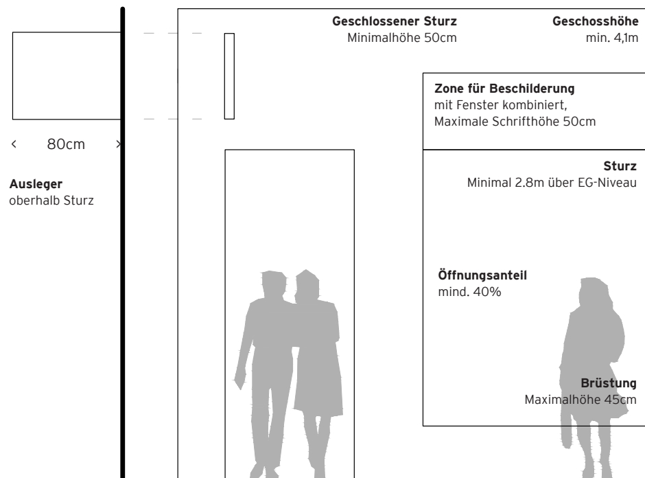
Abb. 233: Regeln für den Sockel in der verlängerten Jaffestraße und im Nahversorgungszentrum
